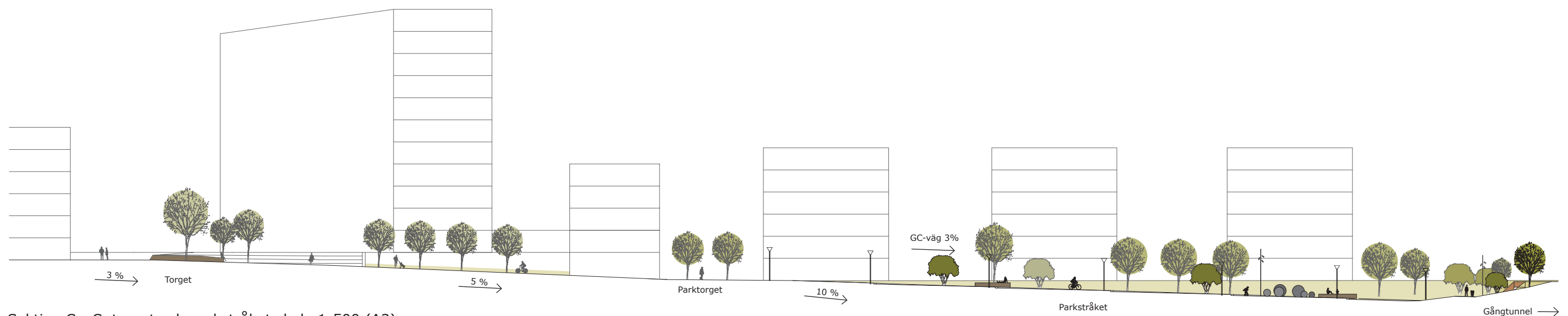
Sektion C - C, torget och parkstråket skala 1:500 (A3)
